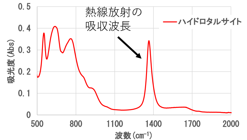
ハイドロタルサイトの吸光度
